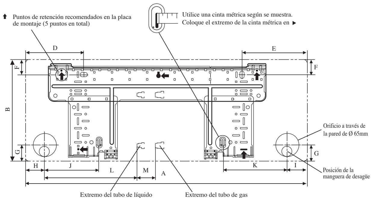
PLACA DE INSTALACIÓN FTXN25/35MV1B
