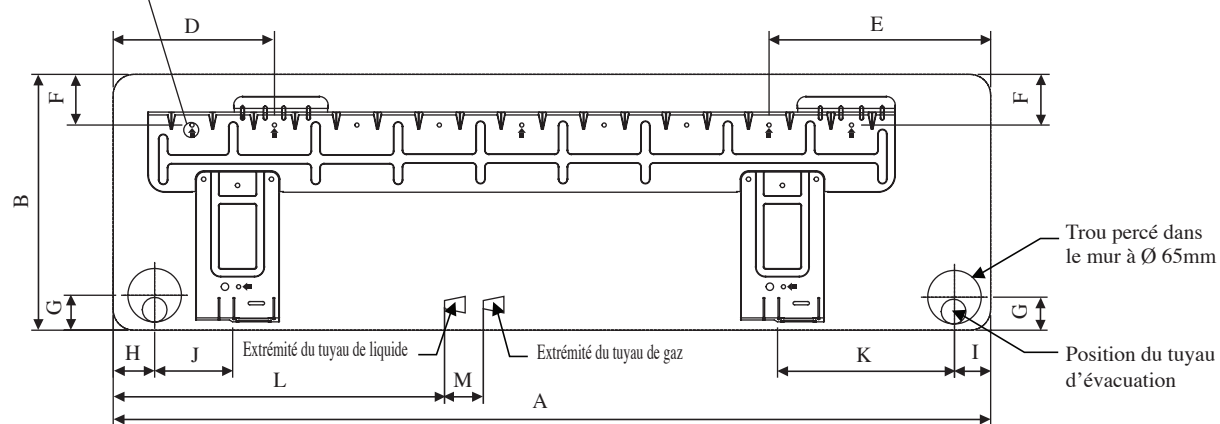
PLAQUE D'INSTALLATION FTXN50/60MV1B
