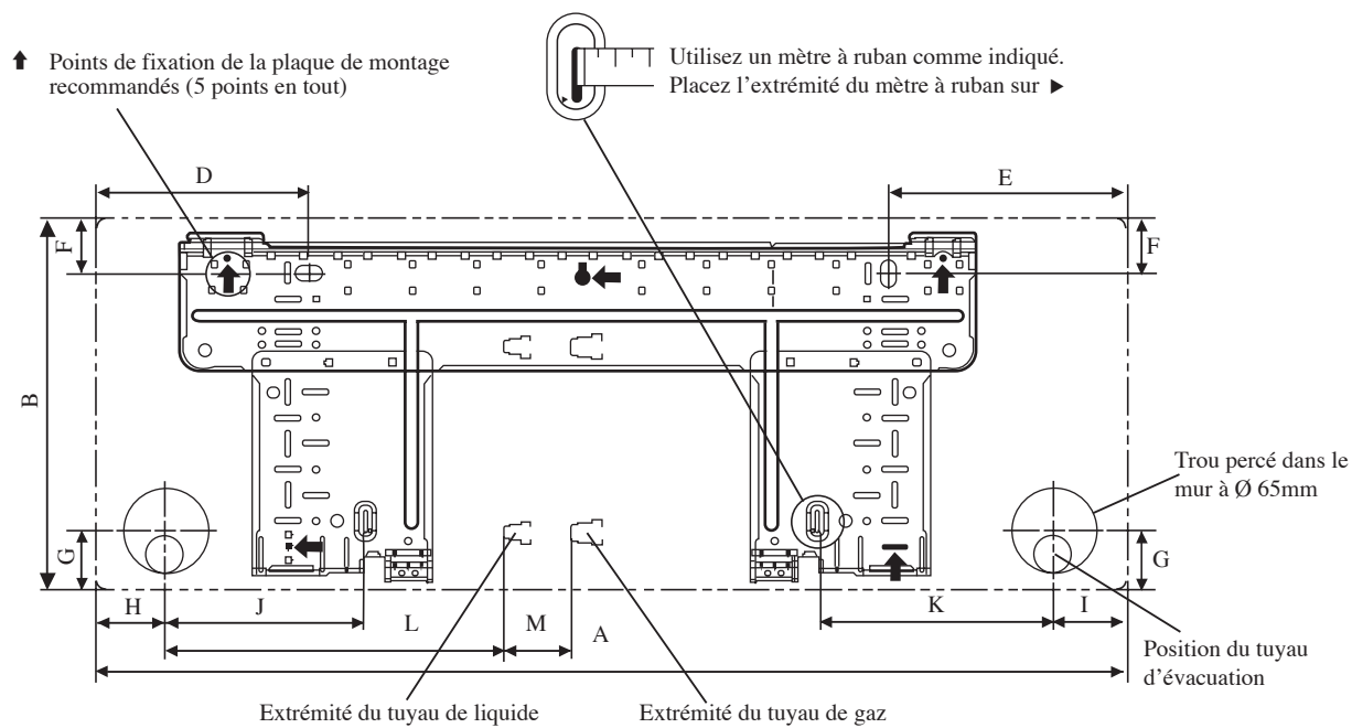
PLAQUE D'INSTALLATION FTXN25/35MV1B
