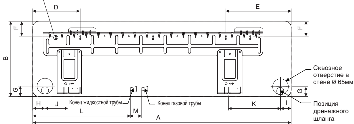
МОНТАЖНАЯ ПЛИТА FTXN50/60MV1B
