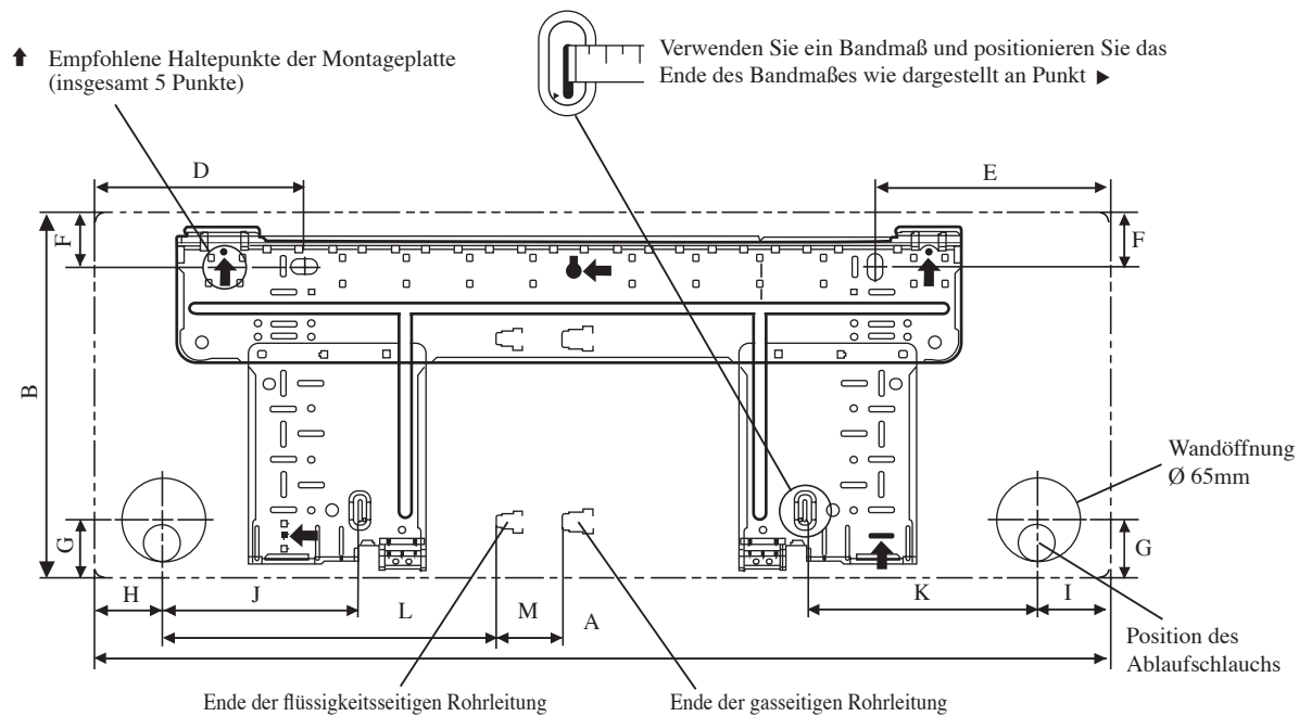
MONTAGEPLATTE FTXN25/35MV1B
