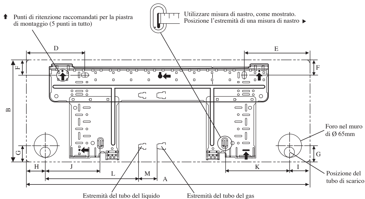
LA STRA DI INSTALLAZIONE FTXN25/35MV1B
