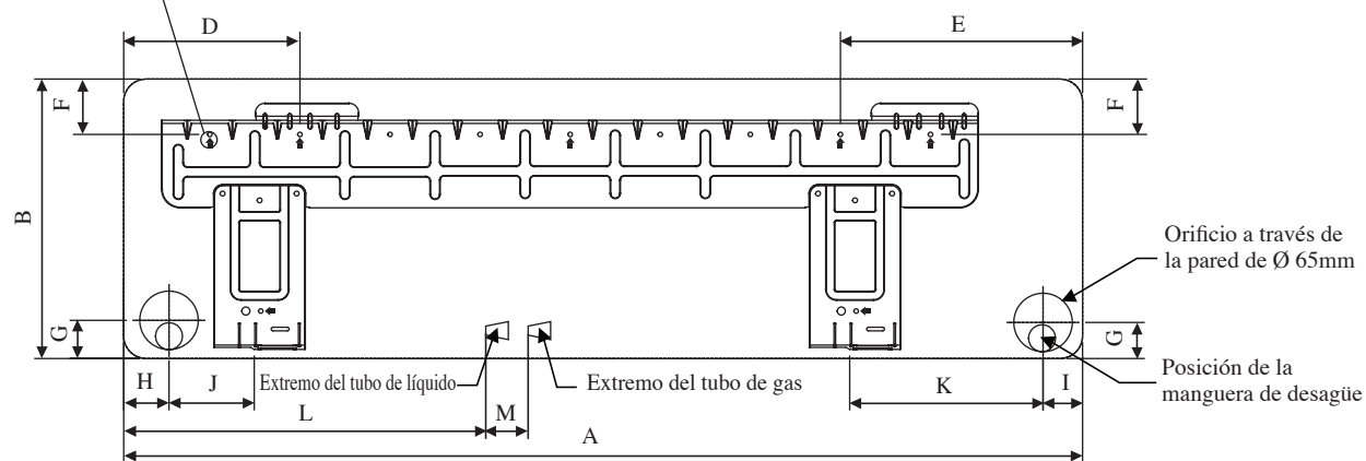
PLACA DE INSTALACIÓN FTXN50/60MV1B
