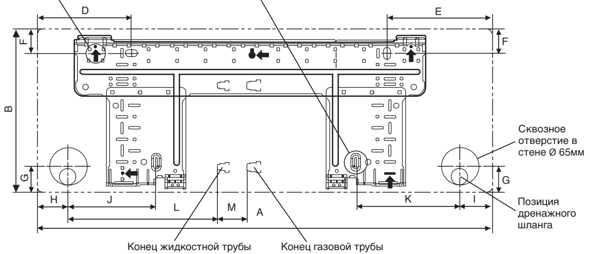
МОНТАЖНАЯ ПЛИТА FTXN25/35MV1B
