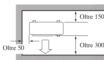
Vista superiore
