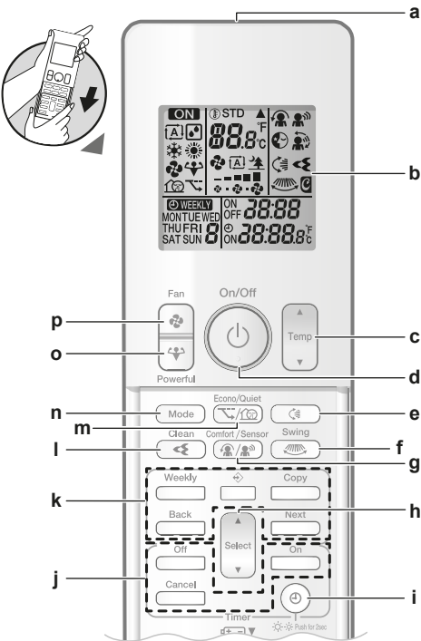
a Transmetteur de signal b Ecran LCD c Bouton de réglage de température d Touche MARCHE/ARRÊT e Touche d'oscillation verticale f Touche d'oscillation horizontale g Débit d'air de confort et bouton de fonctionnement d'œil intelligent h Bouton de sélection i Touche d'horloge et de luminosité de l'écran de l'unité intérieure j Touches de fonctionnement du temporisateur ARRÊT/MARCHE k Touches de fonctionnement de la minuterie hebdomadaire l Touche d'opération (d'épuration d'air) du Flash Streamer m Bouton de fonctionnement silencieux Econo et de l'unité extérieure n Bouton de mode o Bouton de puissance p Touche de ventilateur
